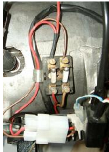
Verkabelung Batterie + Sicherung
